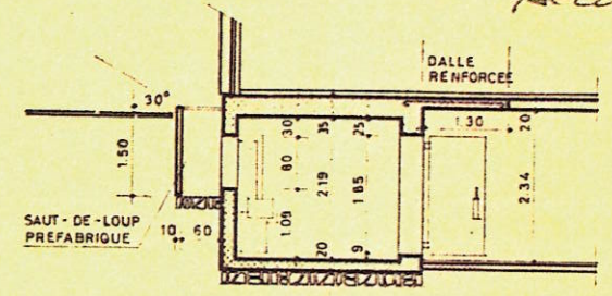
COUPE X-X ECHELLE 1:100
