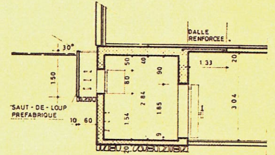
COUPE Y-Y ECHELLE 1:100
